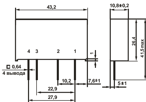
Предельные отклонения между двумя любыми выводами \pm 0,15 мм
