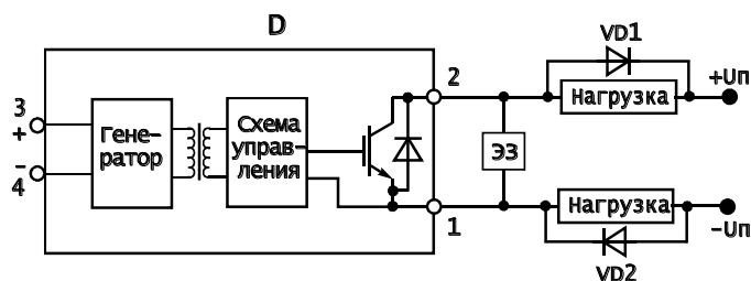
D – модуль VD1, VD2 – диод (устанавливается при индуктивной нагрузке)
