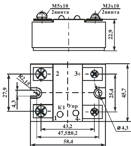
Рисунок 1 – Габаритные и присоединительные размеры модуля
