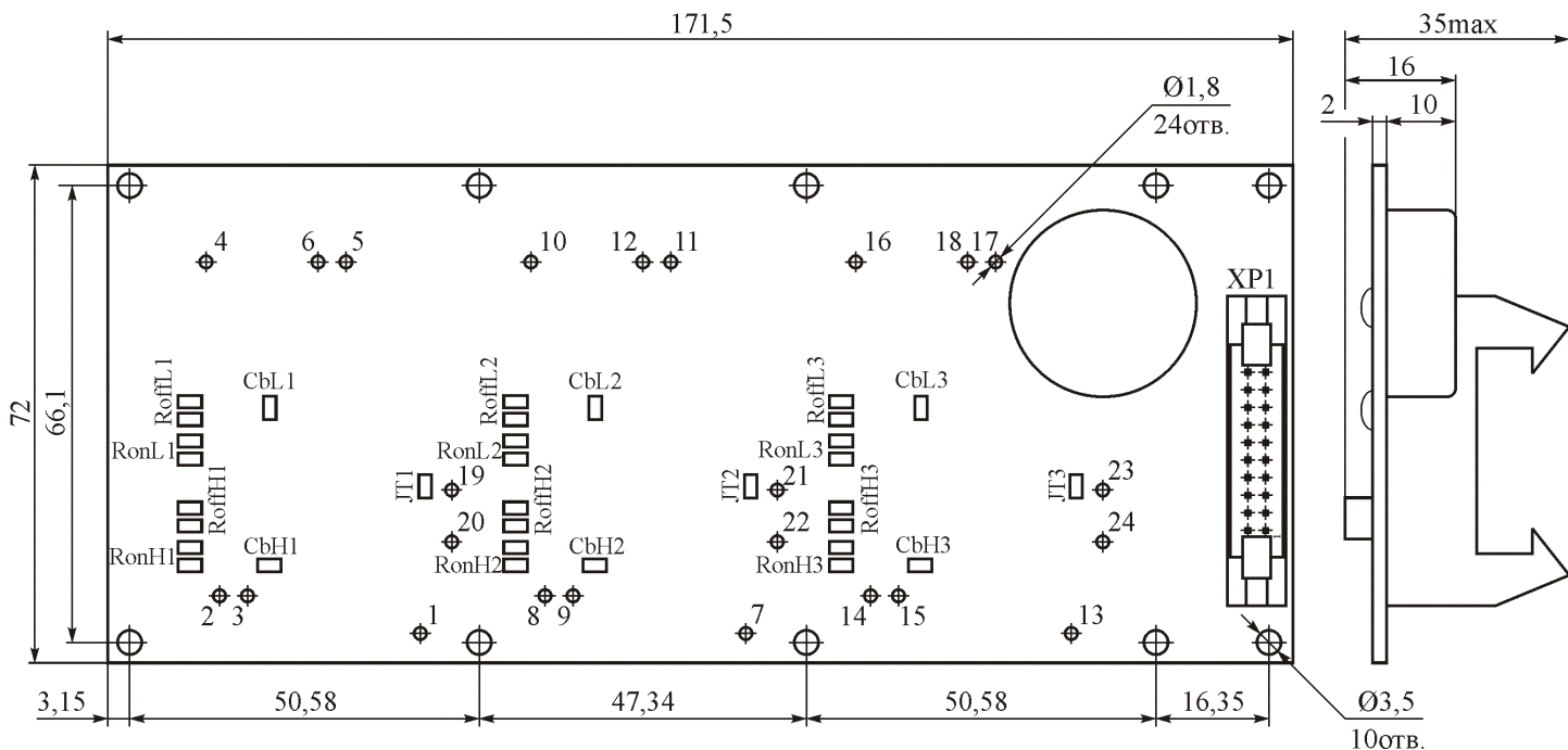
Рисунок 1 – Габаритный чертёж драйвера
