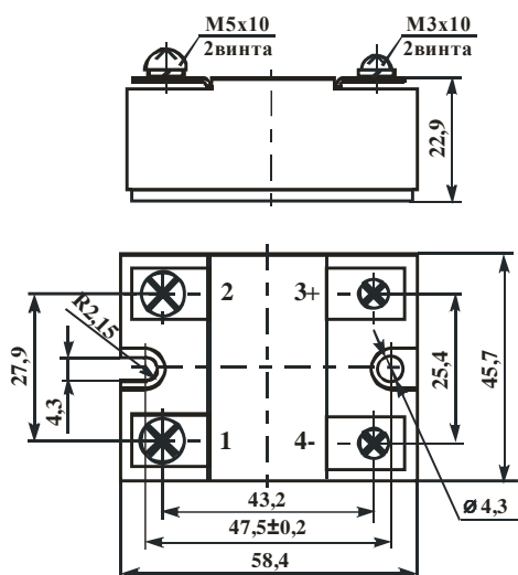
Рисунок 1 – Габаритные и присоединительные размеры модуля
