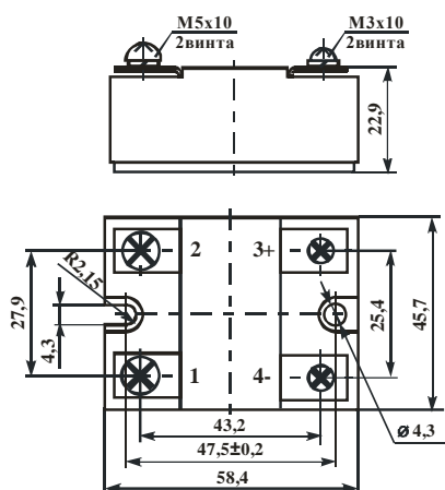
Рисунок 1 – Габаритные и присоединительные размеры модуля
