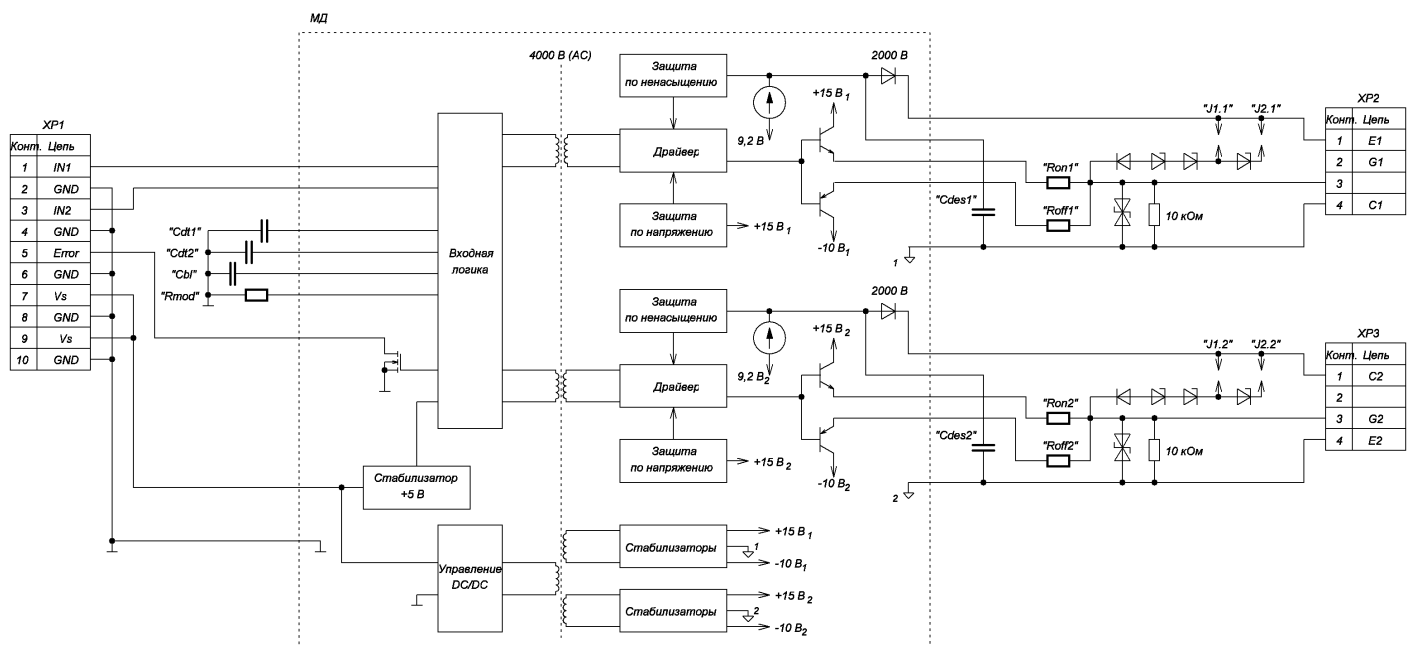
где Cbl – конденсатор настройки длительности блокировки в режиме аварии (см. рисунок 7); Cdt1(2) – конденсаторы настройки длительности «мёртвого» времени на переключение (см. рисунок 5); Cdes – конденсатор настройки задержки срабатывания защиты по ненасыщению (см. рисунок 6); Ron, Roff – резисторы настройки выходного импульсного тока Рисунок 2– Структурная схема драйвера
