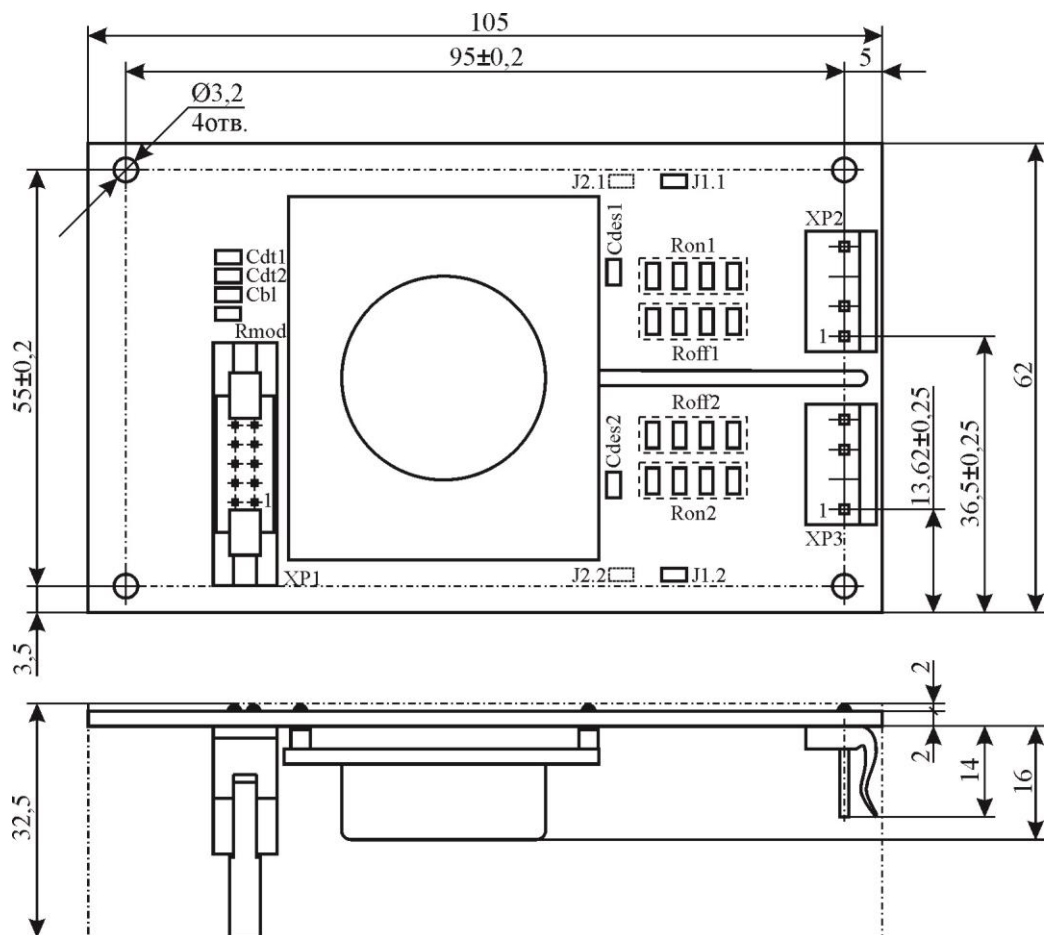
где XP1 – вилка IDCC-10MS (ответная часть – розетка IDC-10); XP2, XP3 – вилки на плату PWL-4 (ответная часть – розетка PHL-4) Рисунок 1 – Габаритный чертеж драйвера
