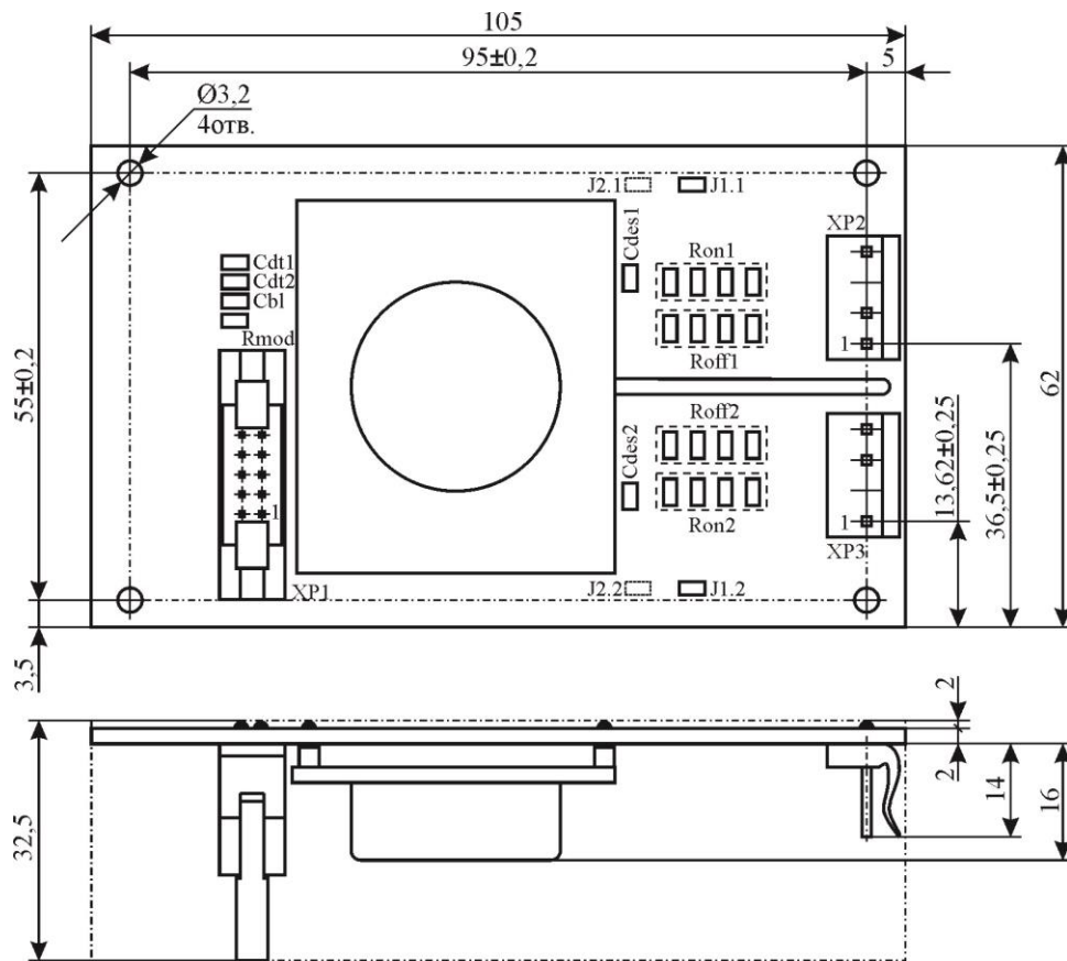
где XP1 – вилка IDCC-10MS (ответная часть – розетка IDC-10); XP2, XP3 – вилки на плату PWL-4 (ответная часть – розетка PHU-4) Рисунок 1 – Габаритный чертеж драйвера
