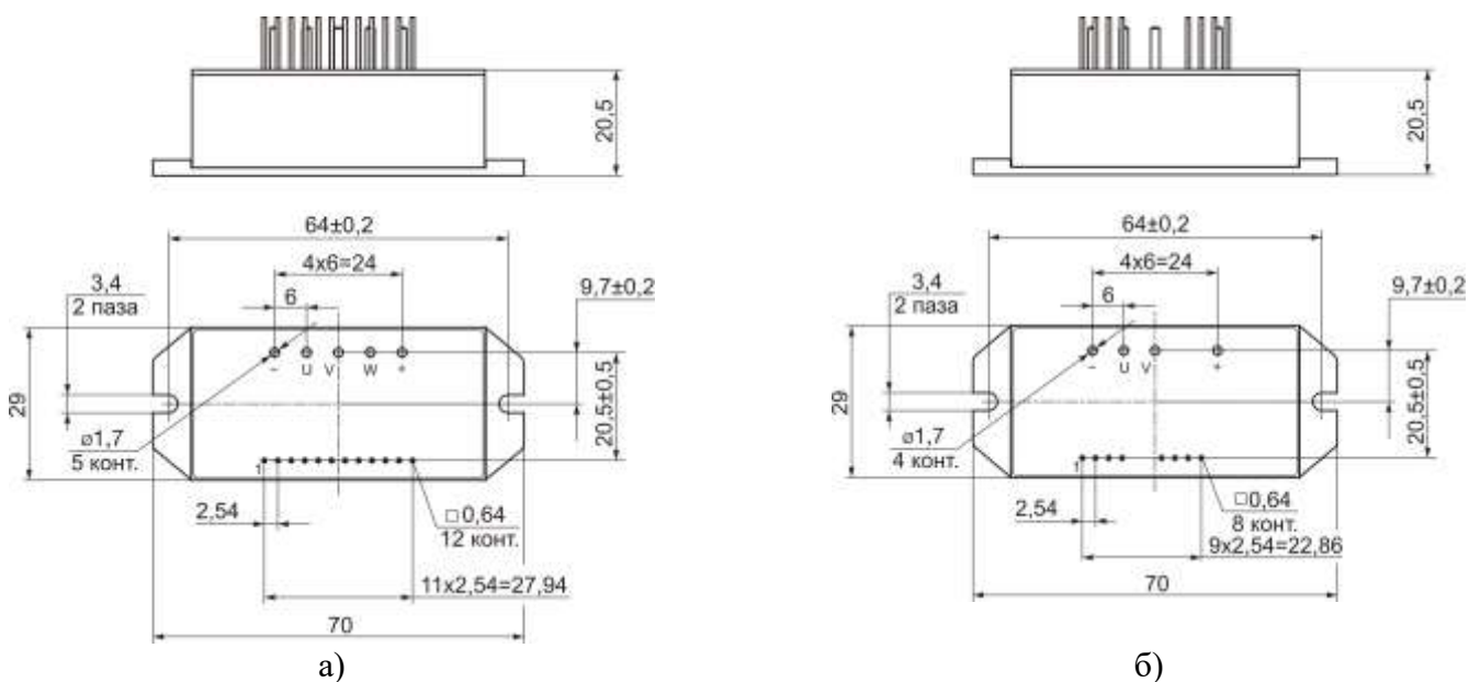
Минимальная высота контактов над корпусом 7 мм Рисунок 2 – Габаритный чертёж модуля
