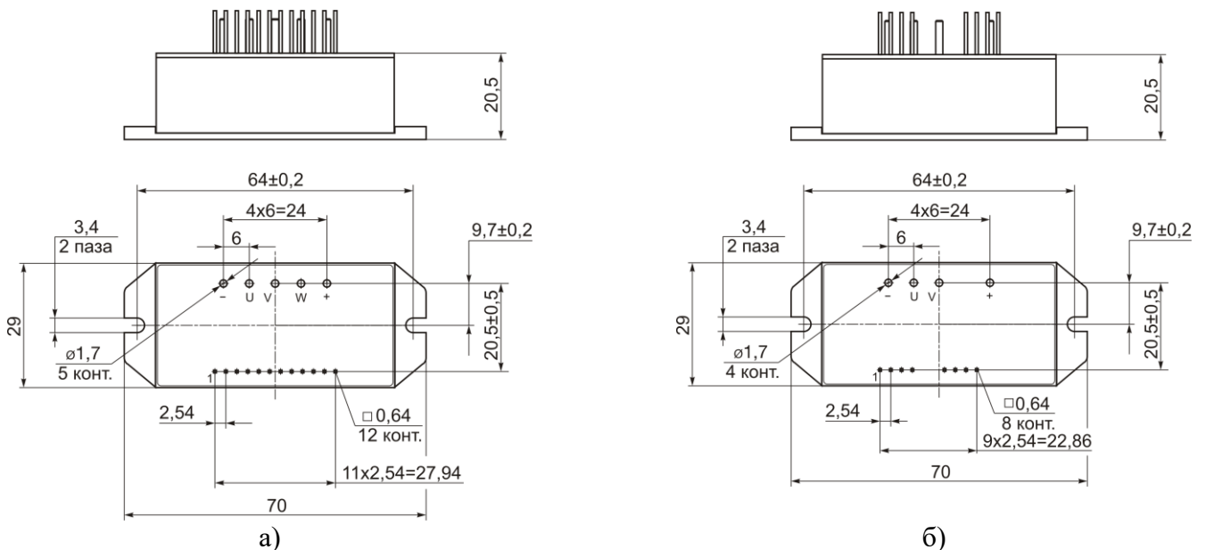
Минимальная высота контактов над корпусом 7 мм Рисунок 2 – Габаритный чертёж модуля
