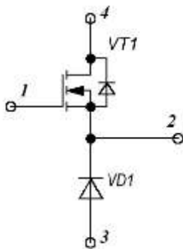
Рисунок 1 – Структурная схема модуля
