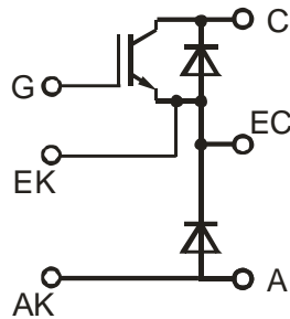
Рисунок 1 – Структурная схема модуля
