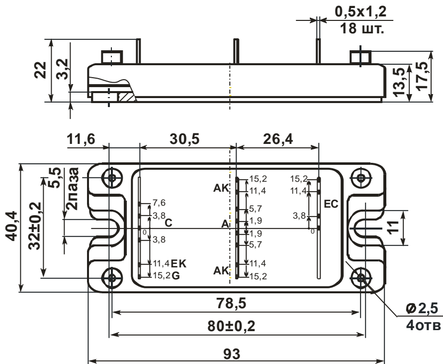
Рисунок 2 – Габаритный чертёж модуля
