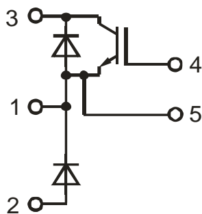
Рисунок 1 – Структурная схема модуля
