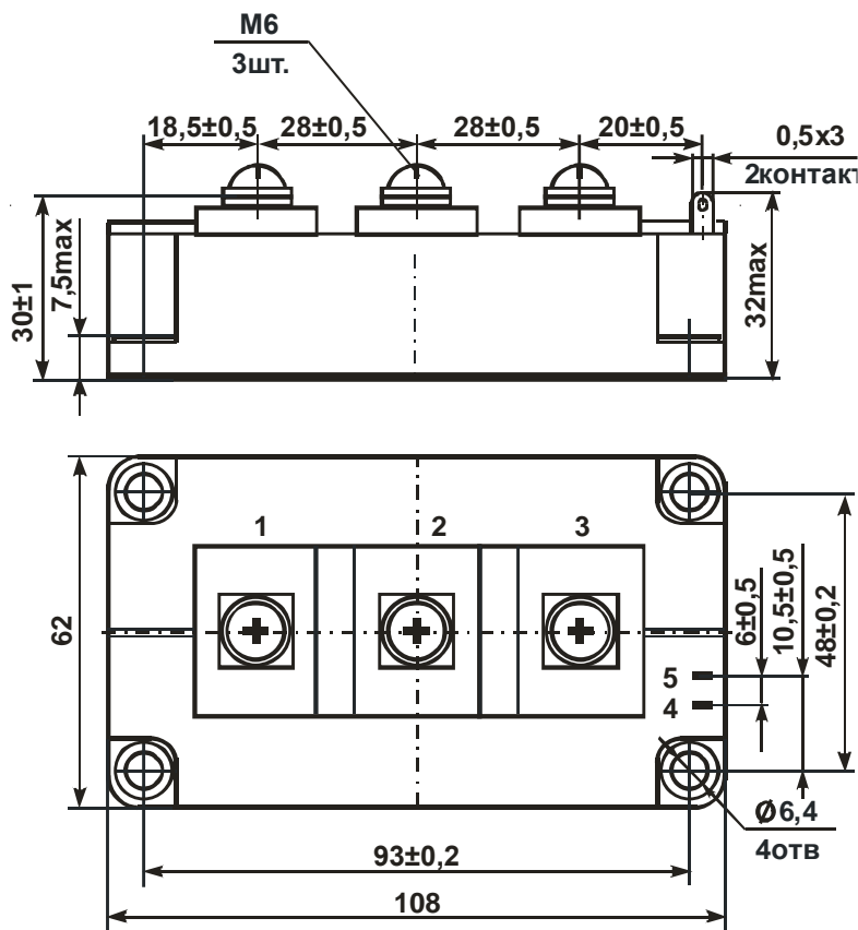
Рисунок 2 – Габаритный чертёж модуля
