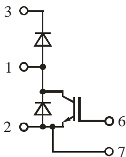
Рисунок 1 – Структурная схема модуля
