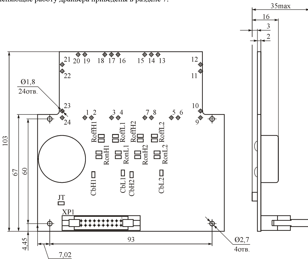
Рисунок 1 – Габаритный чертёж драйвера
