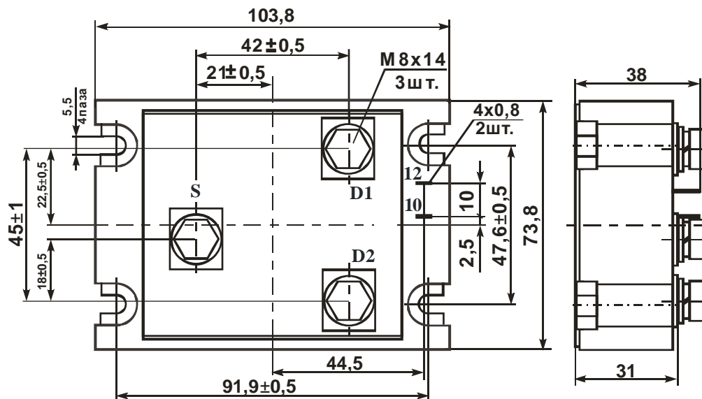
Рисунок 2 – Габаритный чертёж модуля
