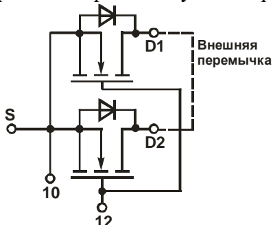
Рисунок 1 – Структурная схема модуля
