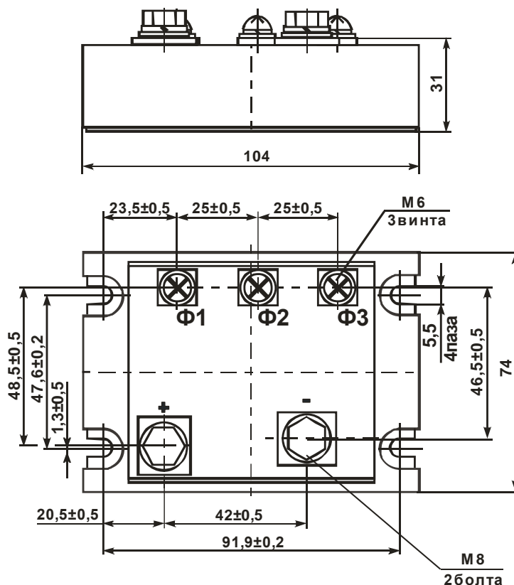
Рисунок 2 – Габаритные и присоединительные размеры модуля
