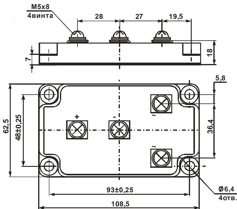
Рисунок 2 – Габаритные и присоединительные размеры модуля
