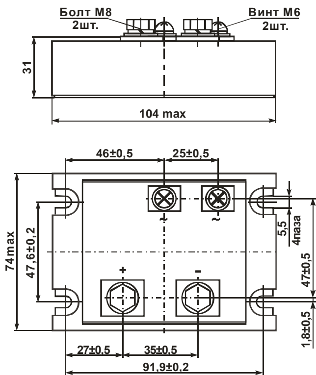
Рисунок 2 – Габаритные и присоединительные размеры модуля
