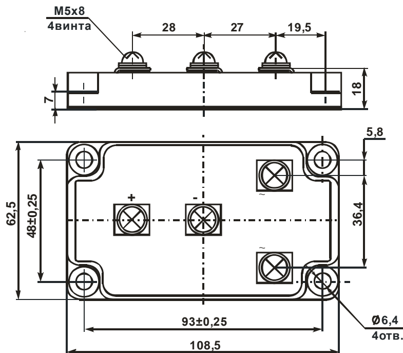
Рисунок 2 – Габаритные и присоединительные размеры
