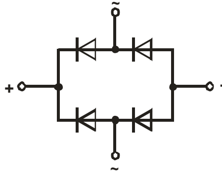
Рисунок 1 – Схема соединения модуля
