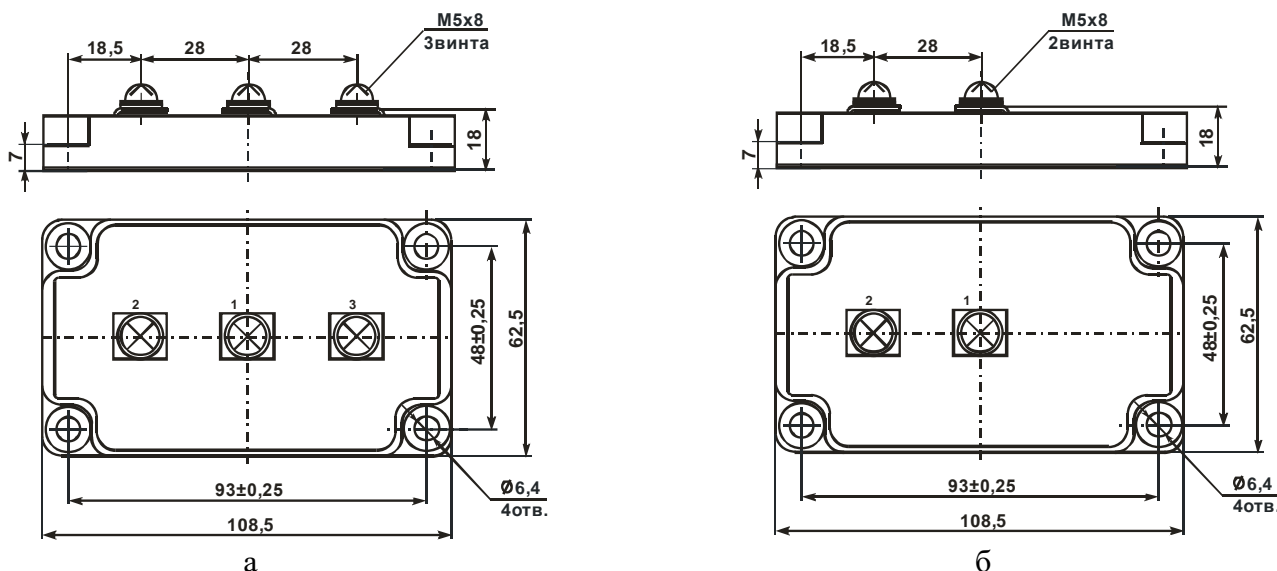
Рисунок 2 – Габаритные и присоединительные размеры
