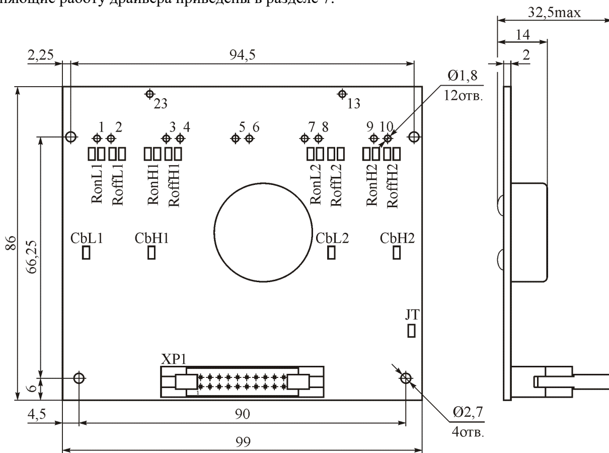
Рисунок 1 – Габаритный чертёж драйвера
