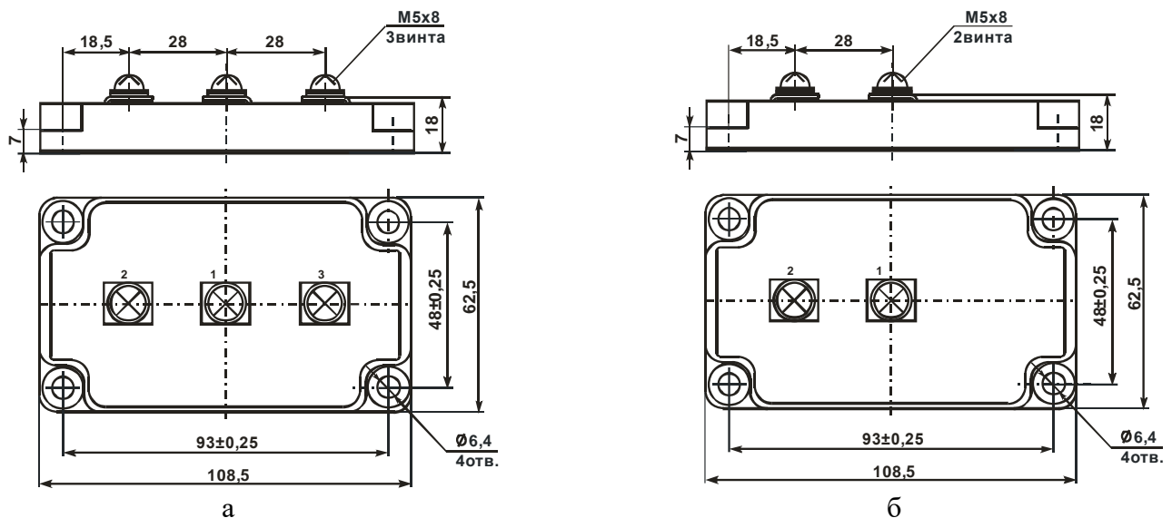
Неуказанные предельные отклонения присоединительных размеров \pm 0,5 мм Рисунок 2 – Габаритные и присоединительные размеры
