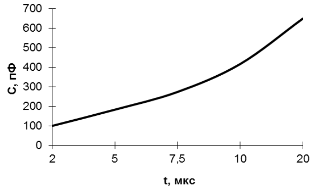
Рисунок 8 – График зависимости длительности задержки включения защиты по насыщению от номинала подстроечной ёмкости C_{mc}
