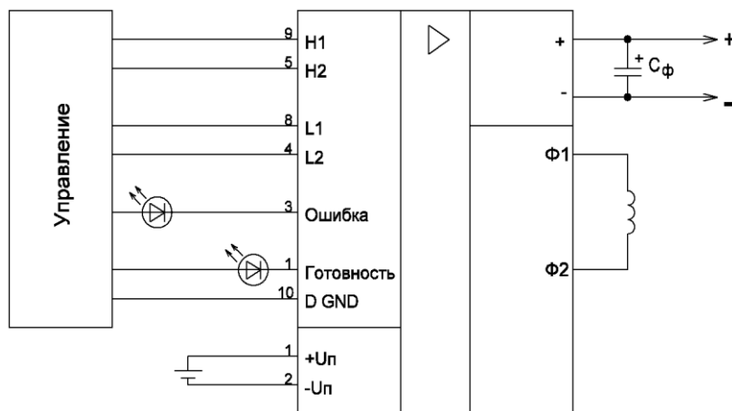
где C_{\phi} – ёмкость фильтра Рисунок 3.4 – Схема включения 1МИ
