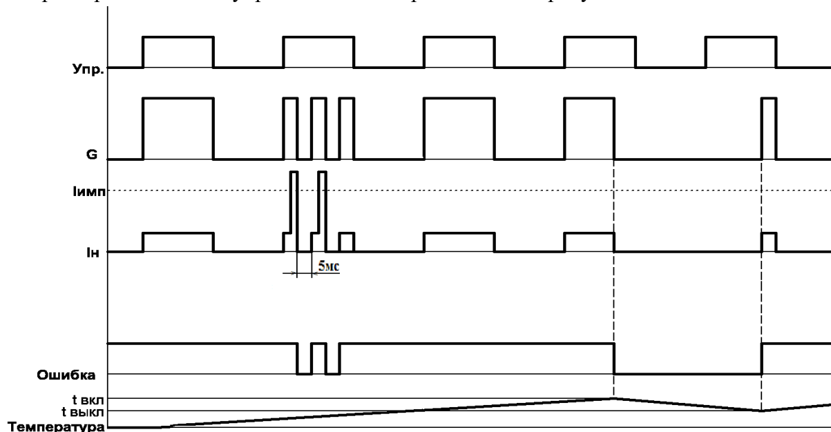
Рисунок 5.1 – Алгоритм работы 1МИ
