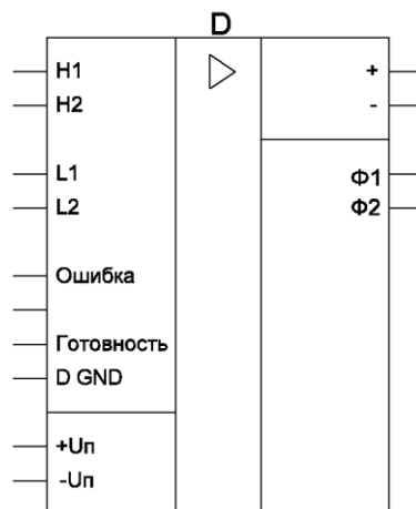
Рисунок 3.3 – Условно-графическое обозначение 1МИ
