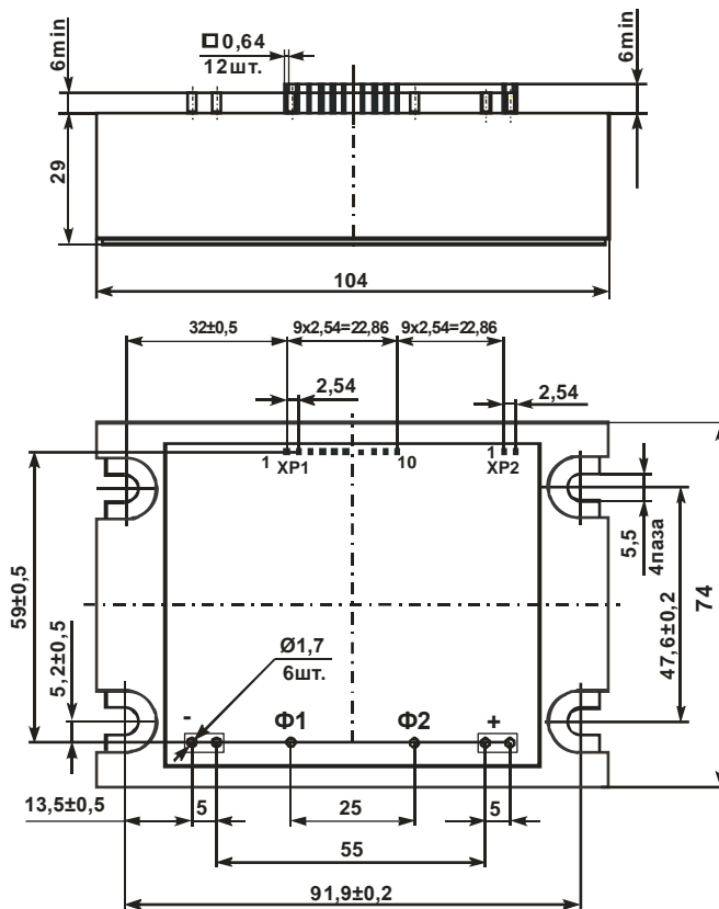
Неуказанные предельные отклонения присоединительных размеров \pm 0,2 мм Рисунок 3.2 – Габаритный чертёж и присоединительные размеры 1МИ
