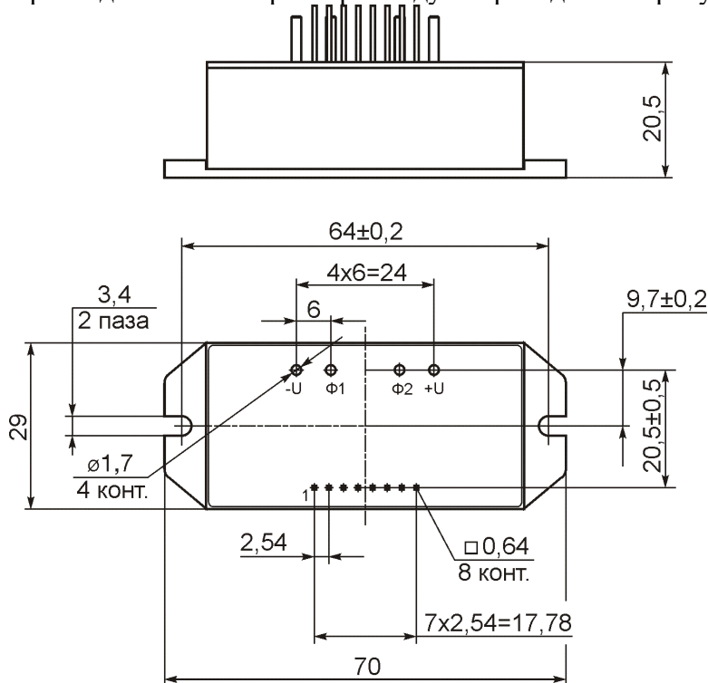
Рисунок 6.1 - Габаритные и присоединительные размеры модуля
