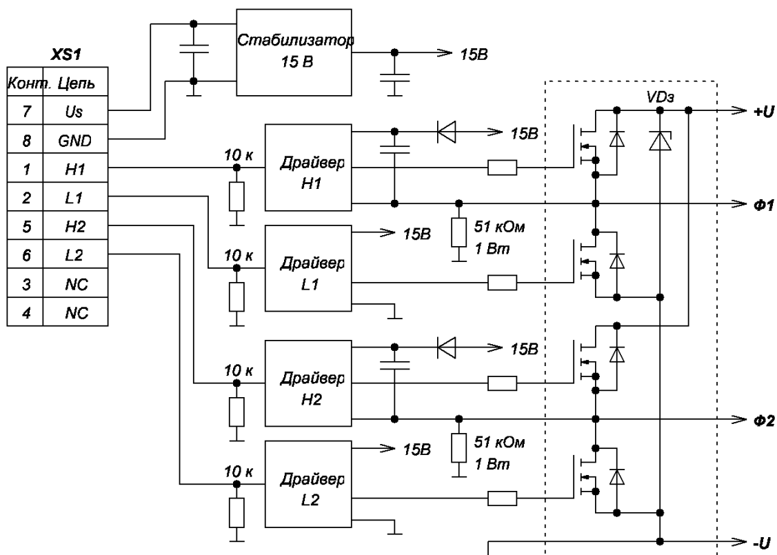
Рисунок 1.1 – Структурная схема модуля
