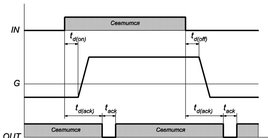
Рисунок 4 – Диаграмма штатной работы драйвера
