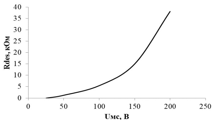
Рисунок 10 – График зависимости напряжения срабатывания защиты по насыщению от номинала резистора R_{des}
