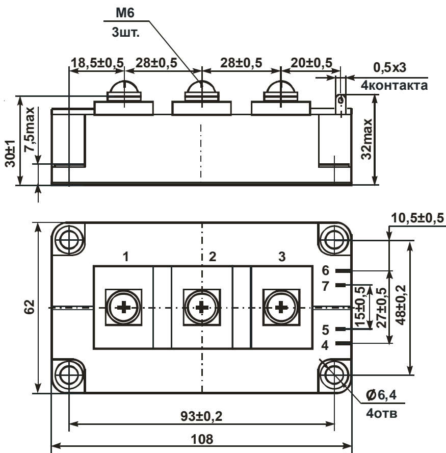
Рисунок 2 – Габаритный чертёж модуля
