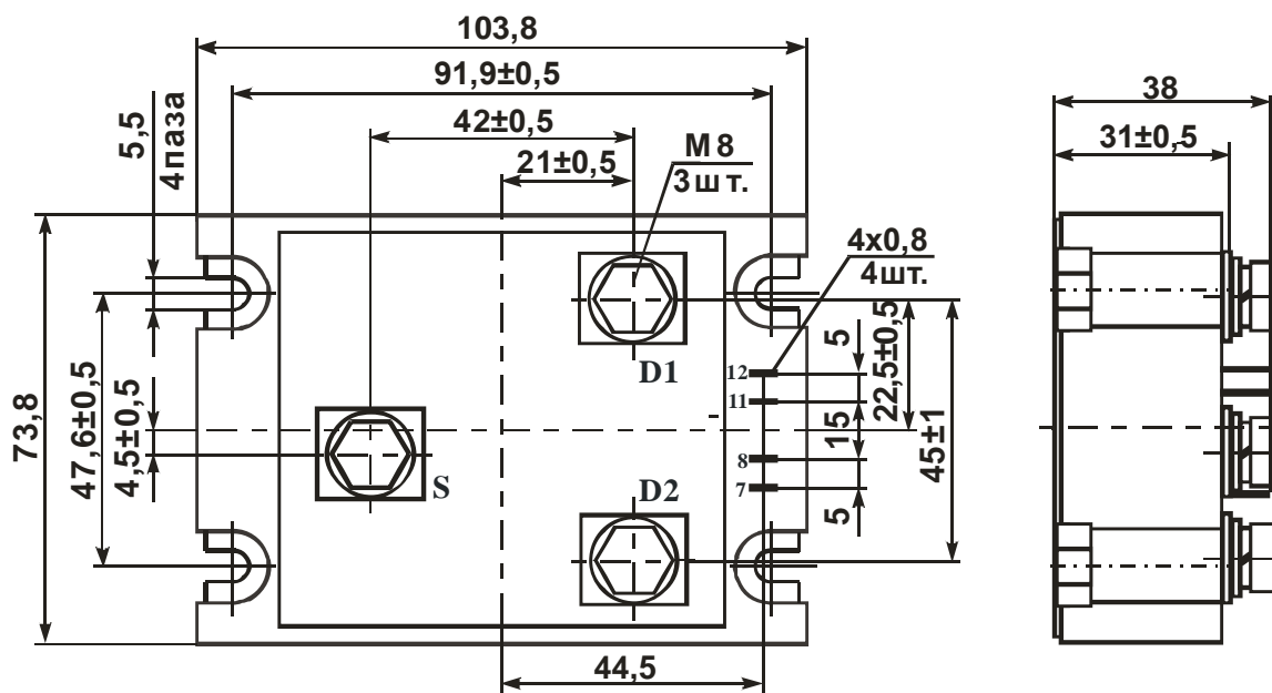
Рисунок 2 – Габаритный чертёж модуля
