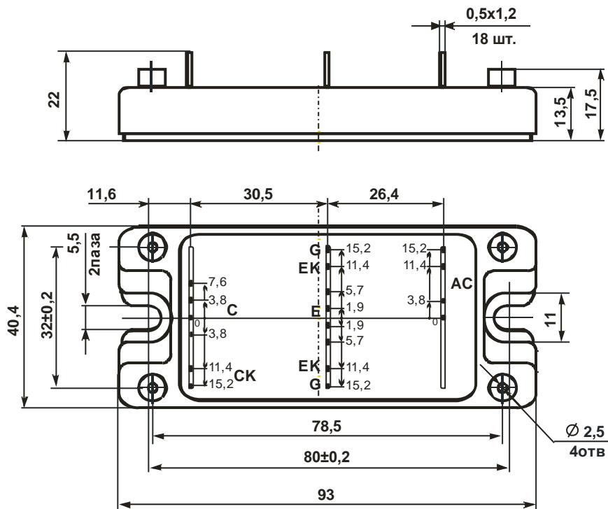
Рисунок 2 – Габаритный чертёж модуля
