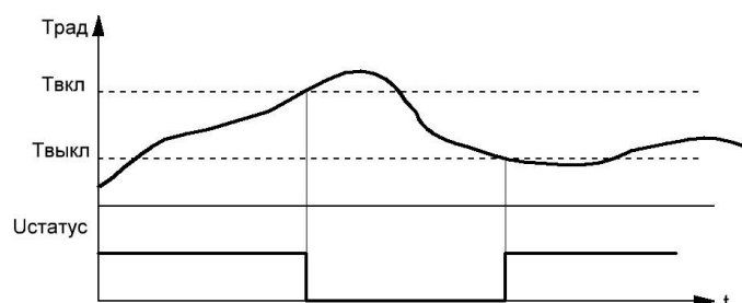
Рисунок 3 – Диаграмма функционирования температурной сигнализации
