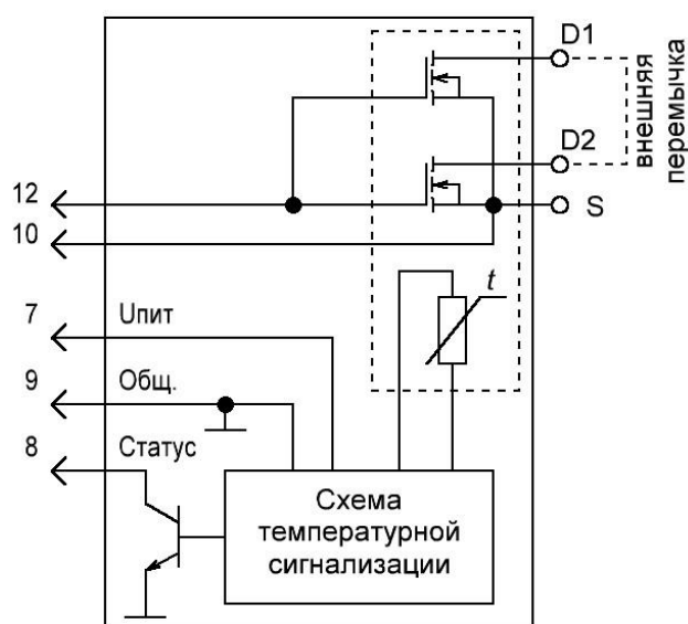
Рисунок 1 – Электрическая схема соединения элементов модуля
