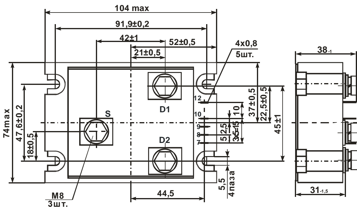
Рисунок 2 – Габаритный чертёж модуля
