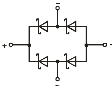
Рисунок 1 – Схема соединения модуля
