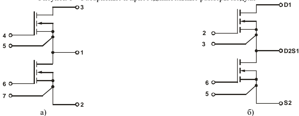
а) б) Рисунок 2 – Электрическая схема внутренних соединений модуля
