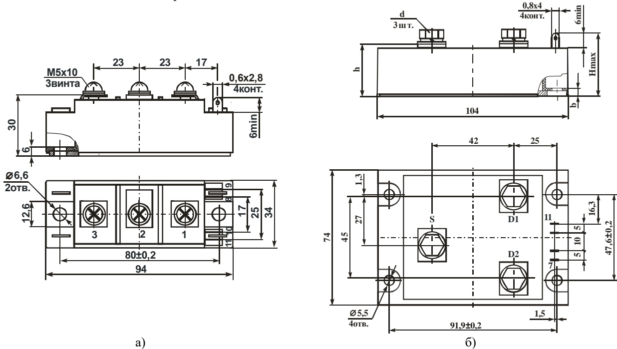
а) б) Неуказанные предельные отклонения присоединительных размеров \pm 0,5 мм Рисунок 1 – Габаритные и присоединительные размеры модуля
