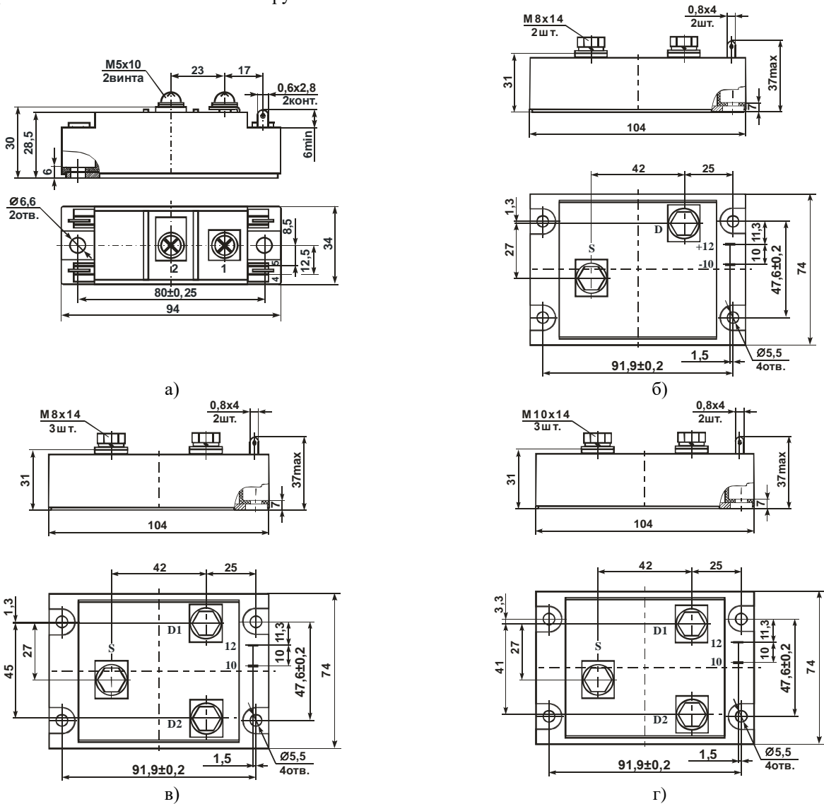
Неуказанные предельные отклонения присоединительных размеров ±0,5 мм Рисунок 1 – Габаритные и присоединительные размеры модуля
