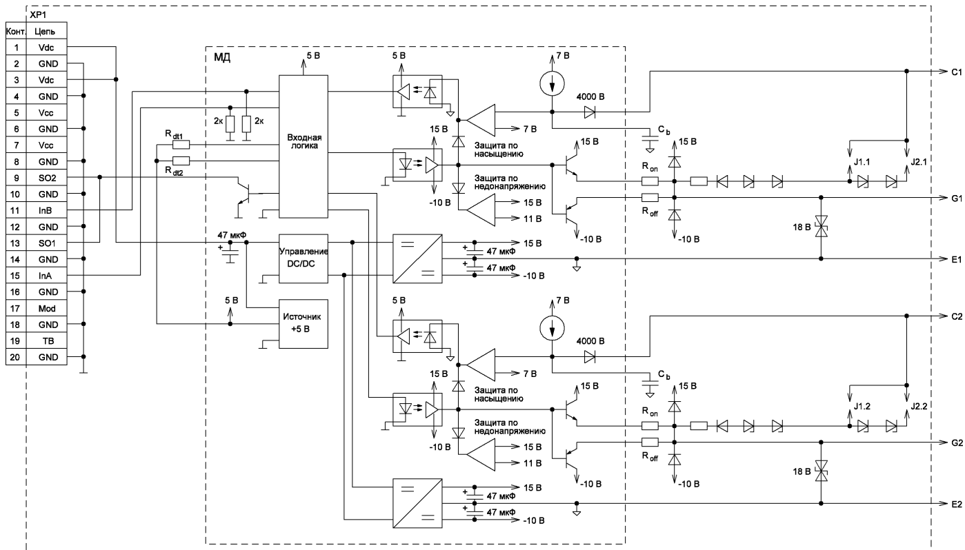
Рисунок 2– Функциональная схема драйвера
