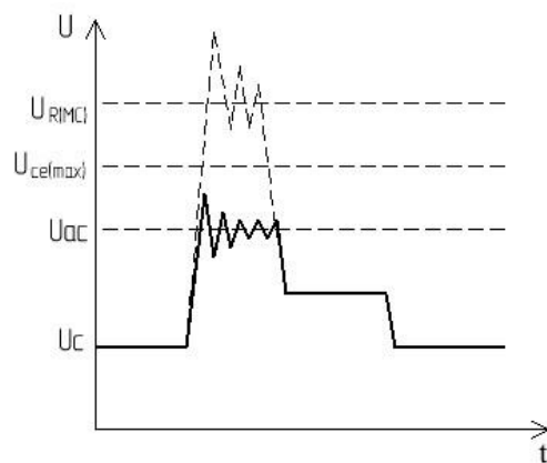
Рисунок 12 – График работы драйвера при срабатывании защиты от перенапряжения коллектор-эмиттер управляемого транзистора где U_{ce} – напряжение срабатывания защиты от перенапряжения; U_{ce(max)} – максимальное напряжение коллектор-эмиттер силового транзистора, U_r(ms) – максимально допустимое обратное напряжение на выводе коллектора драйвера
