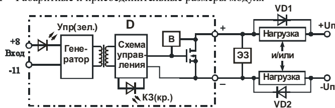
D – модуль; B – блок активной защиты (обеспечивает ограничение напряжения на стоке транзистора на уровне не более U_{огр} ); VD1, VD2 – диод (устанавливается при индуктивной нагрузке); ЭЗ – элемент защиты.
