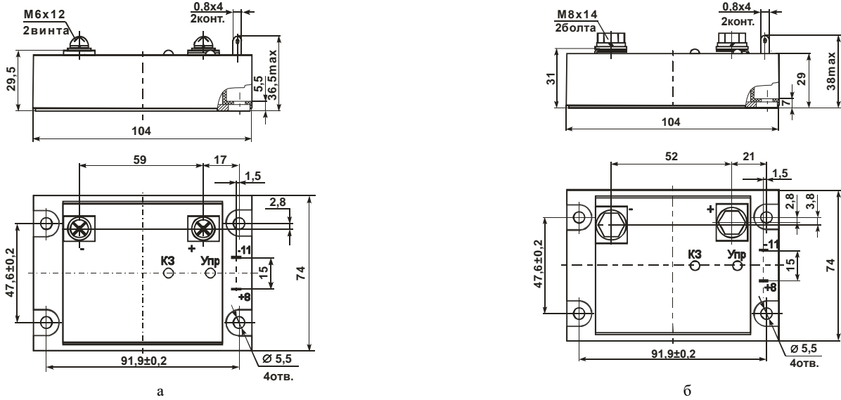
а б Неуказанные предельные отклонения присоединительных размеров \pm 0,5 мм Рисунок 1 – Габаритные и присоединительные размеры модуля
