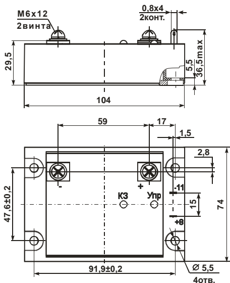
Рисунок 1 – Габаритные и присоединительные размеры модуля
