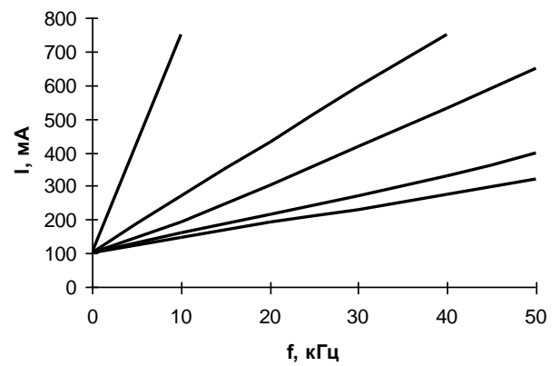
Рисунок 5 – График зависимости тока потребления от частоты сигнала под нагрузкой (с затворным резистором 5 Ом) для ёмкостей нагрузки 10 нФ, 25 нФ, 50 нФ, 100 нФ и 250 нФ
