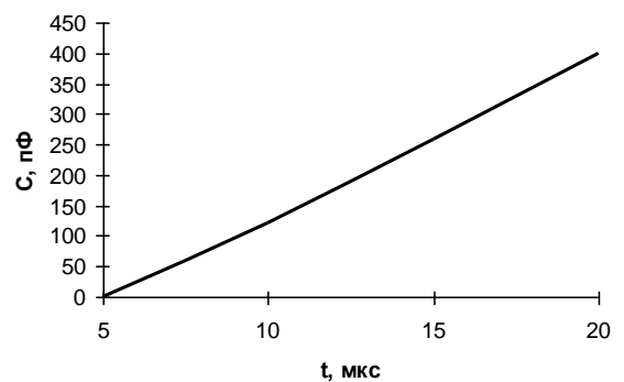
Рисунок 9 – График зависимости длительности задержки включения защиты по насыщению от ёмкости
