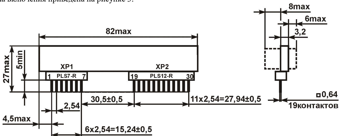
Рисунок 1 – Габаритный чертёж драйвера
