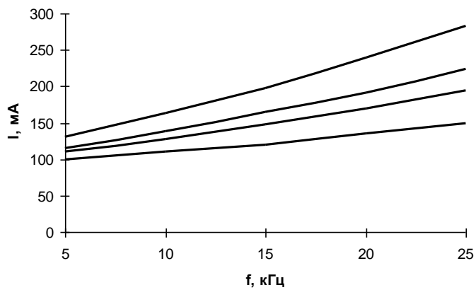
Рисунок 6 – График зависимости тока потребления драйвером от частоты сигнала управления под нагрузкой (с затворным резистором 1 Ом) для ёмкостей нагрузки 10 нФ, 25 нФ, 50 нФ, 100 нФ
