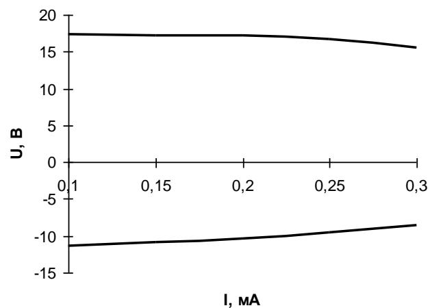
Рисунок 7 – График зависимости амплитуды напряжений на затворе управляемого транзистора от тока потребления драйвера
