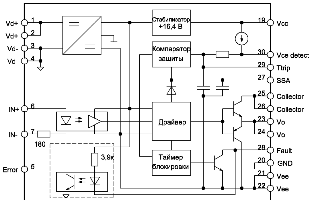
Где пунктиром выделен блок, входящий только в состав МД1120П-А1 Рисунок 2 – Функциональная схема драйвера
