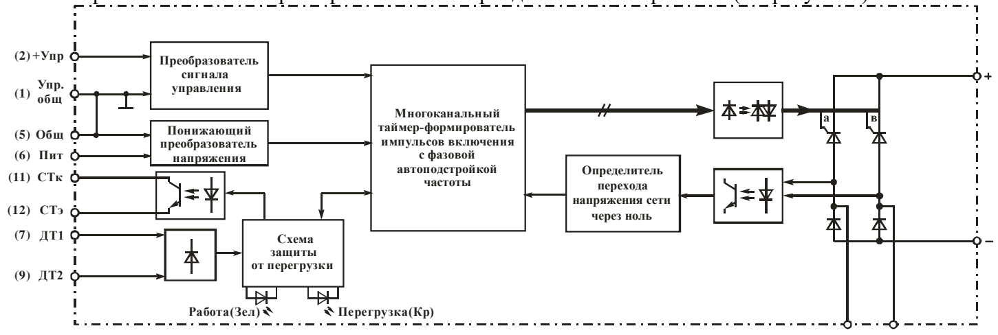
Рисунок 1 – Функциональная схема модуля
