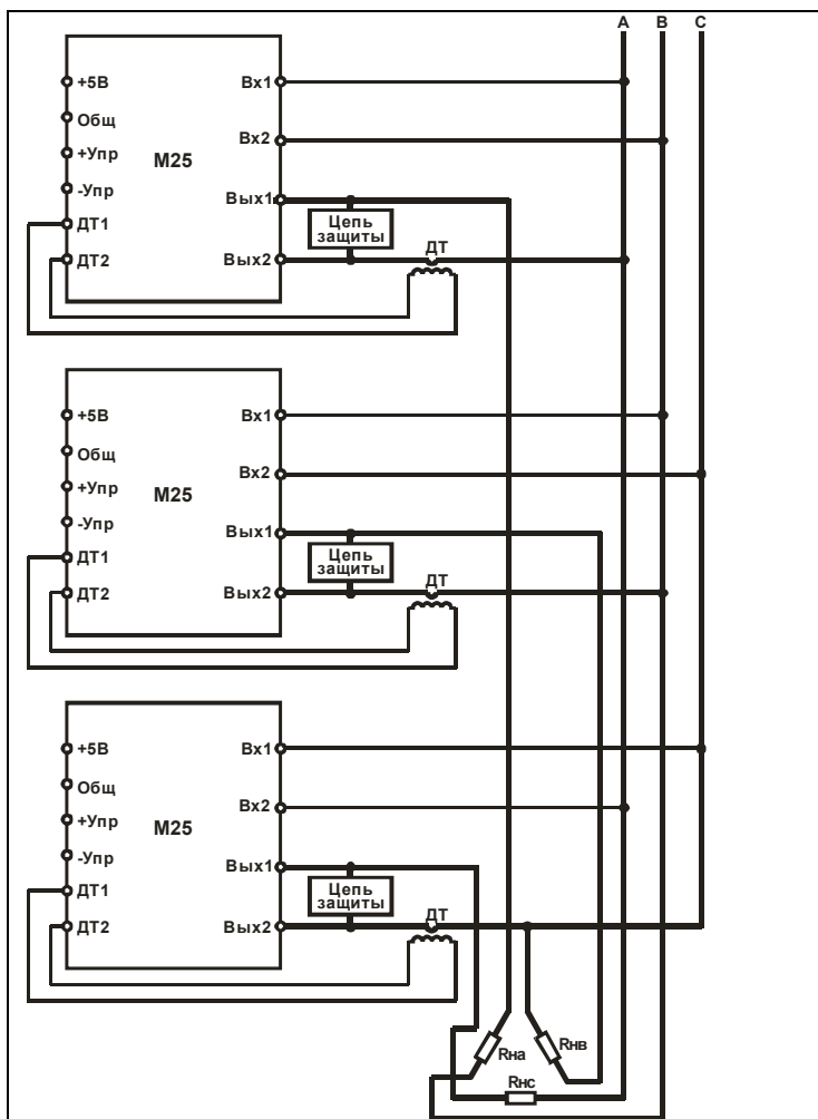
Рисунок 7а – Пример схемы трехфазного регулятора мощности на М25 (открытое соединение в «треугольник» (шестипроводное соединение))
