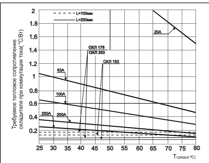
Рисунок 8г – При скорости охлаждающего воздуха 12 м/с
