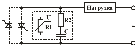
Рисунок 5 – Защитная цепь
