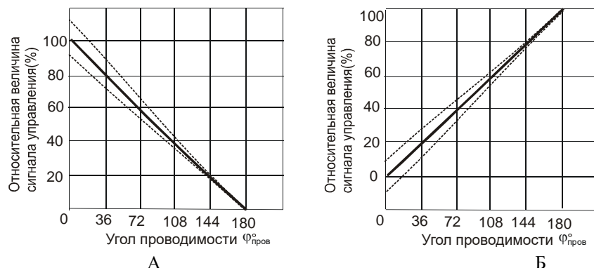
А – 100% сигнала управления соответствуют минимальной мощности; Б – 100% сигнала управления соответствуют максимальной мощности
