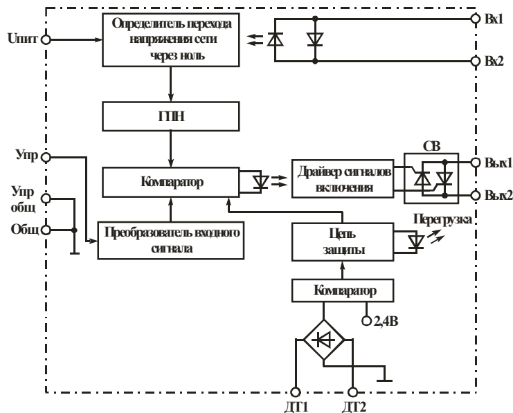
Рисунок 1 – Функциональная схема модуля
