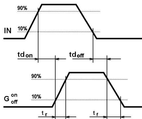
где IN – входной сигнал управления; G – сигнал на затворе управляемого транзистора Рисунок 12 – Диаграмма, поясняющая временные параметры драйвера
