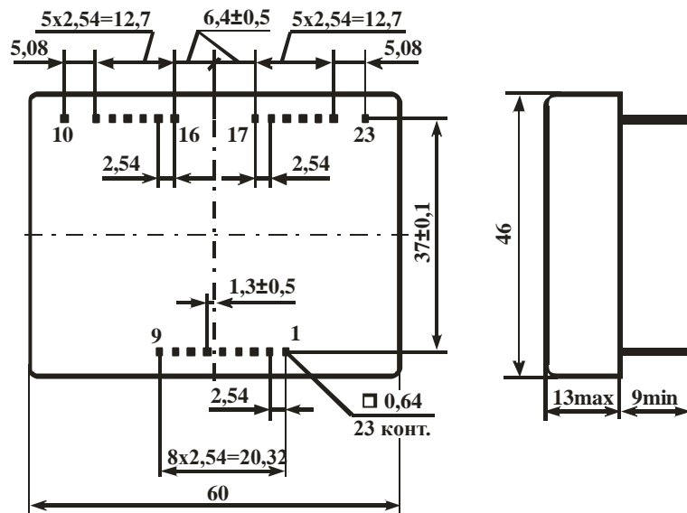
Рисунок 1 – Габаритный чертёж драйвера
