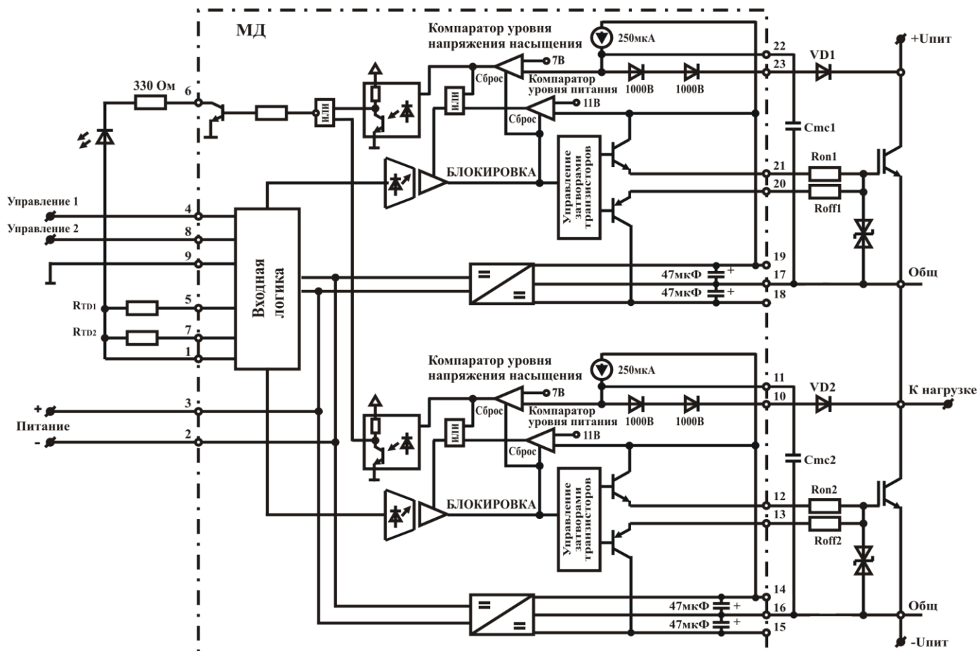
Рисунок 2 – Функциональная схема и схема включения драйвера
