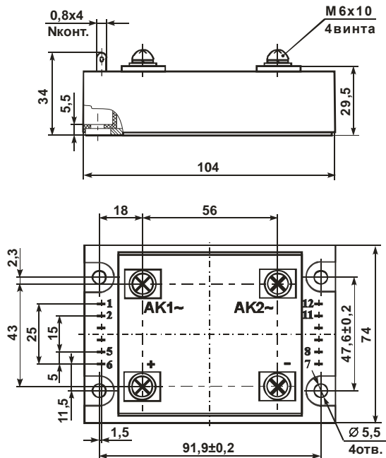
Неуказанные отклонения присоединительных размеров ±0,5мм Рисунок 1 – Габаритные и присоединительные размеры модулей
