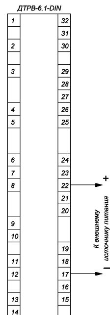
Рисунок 7 – Схема питания внешнего каскада от внешнего источника питания
