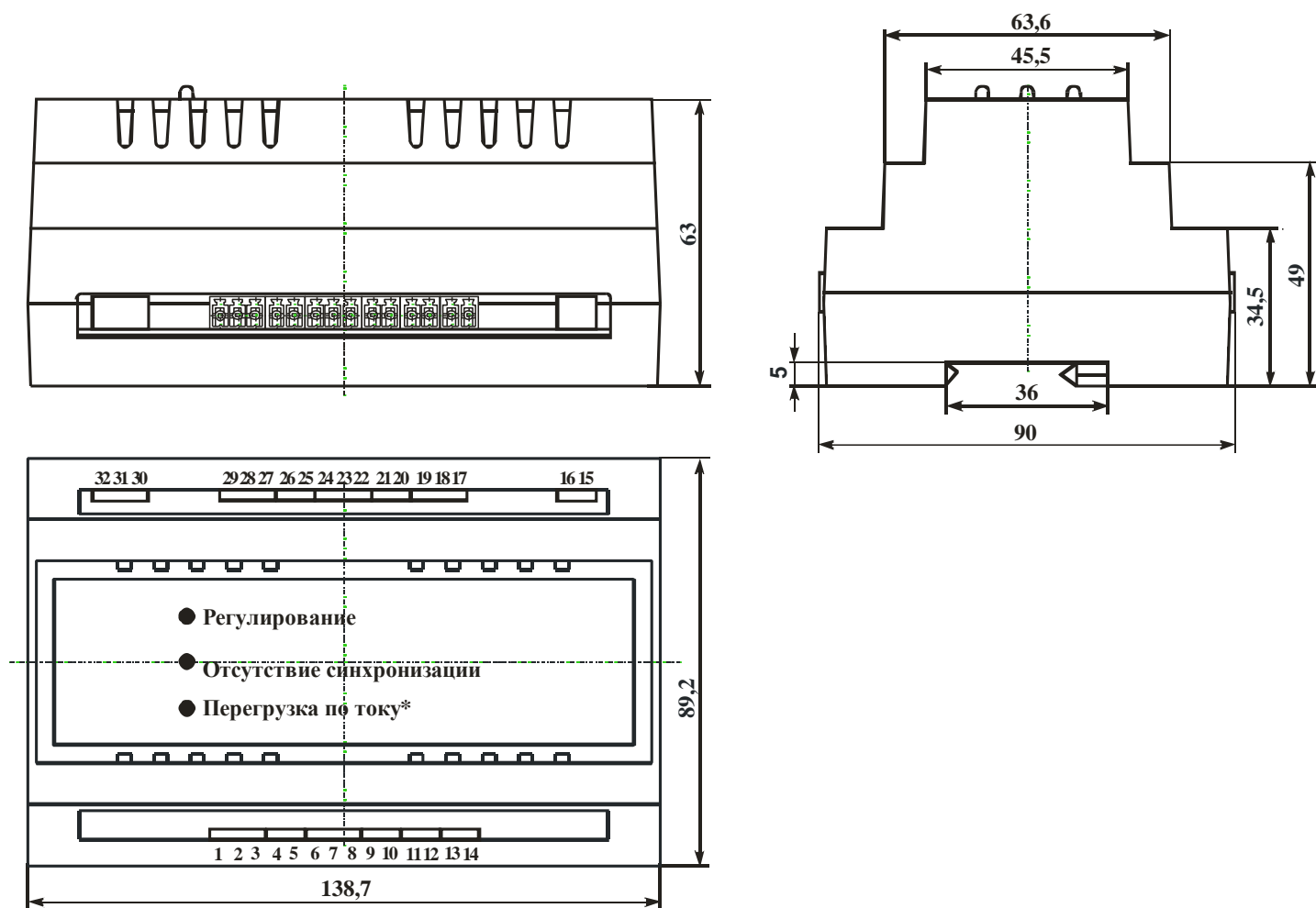
Рисунок 3 – Габаритные и присоединительные размеры
