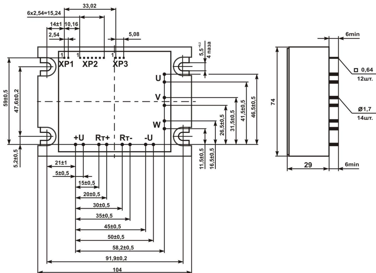
Рисунок 4 – Габаритный чертёж и присоединительные размеры модуля
