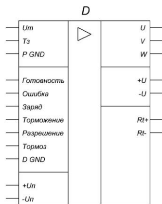
Рисунок 1 – Структурная схема модуля
