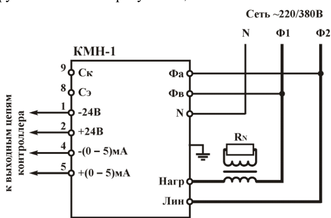
Рисунок 4 – Схема включения КМН-1 в однофазном режиме «Фаза – Фаза» (нагрузка активная или активно-индуктивная рассчитана на линейное напряжение сети ~380 В)
