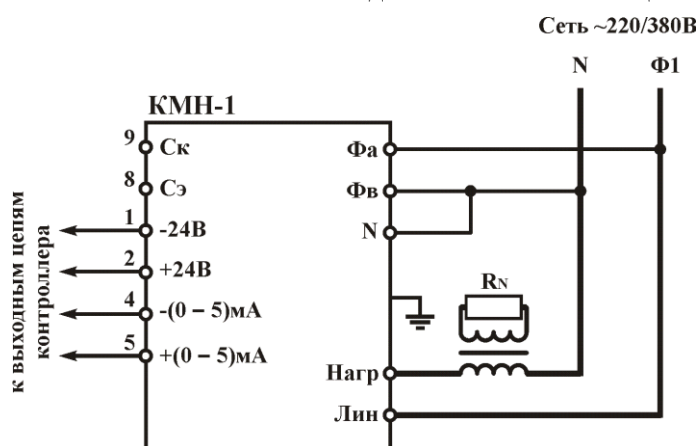
Рисунок 3 – Схема включения КМН-1 в однофазном режиме «Фаза – Ноль» (нагрузка активная или активно-индуктивная рассчитана на фазное напряжение сети ~220 В)
