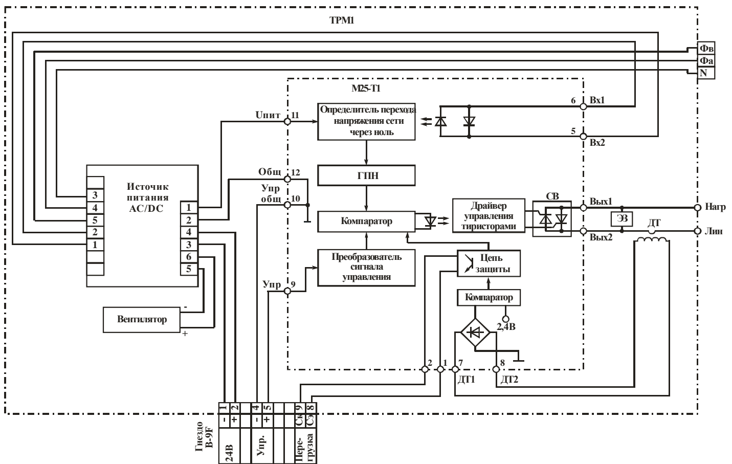
Рисунок 1 – Схема электрическая функциональная
