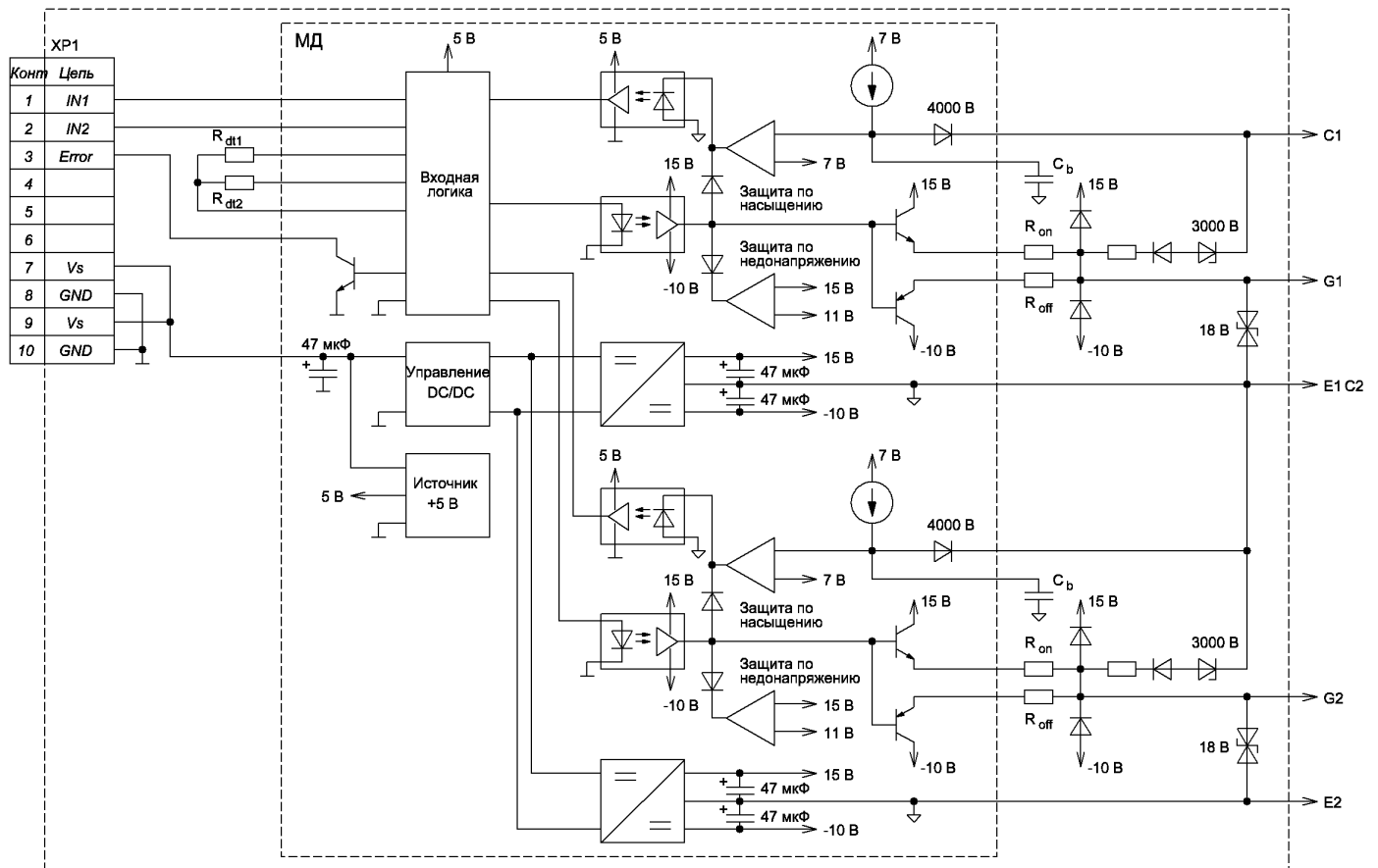
где XP1 – вилка IDCC-10MS; ответная часть – розетка IDC-10; Рисунок 2– Функциональная схема драйвера
