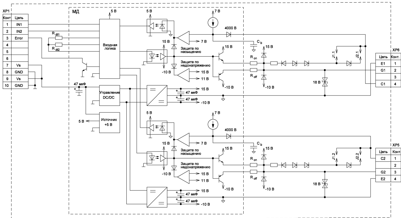
где XP1 – вилка IDCC-10MS, ответная часть – розетка IDC-10; XP5, XP6 – вилки на плату PWL-4, ответная часть – розетка PNU-4 Рисунок 2– Функциональная схема драйвера
