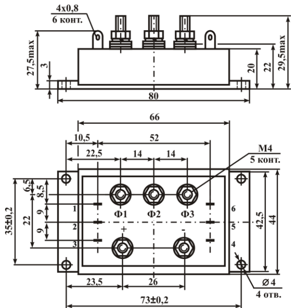
Рисунок 1 – Габаритные и присоединительные размеры модулей
