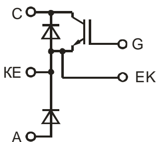
Рисунок 1 – Структурная схема модуля
